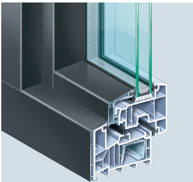
AluFusion System, flächenversetzt Fenstersystem mit 88 mm Bautiefe, PVC-Flügelprofil und Alu-Funktionsprofil in gleitender Verbindung.
